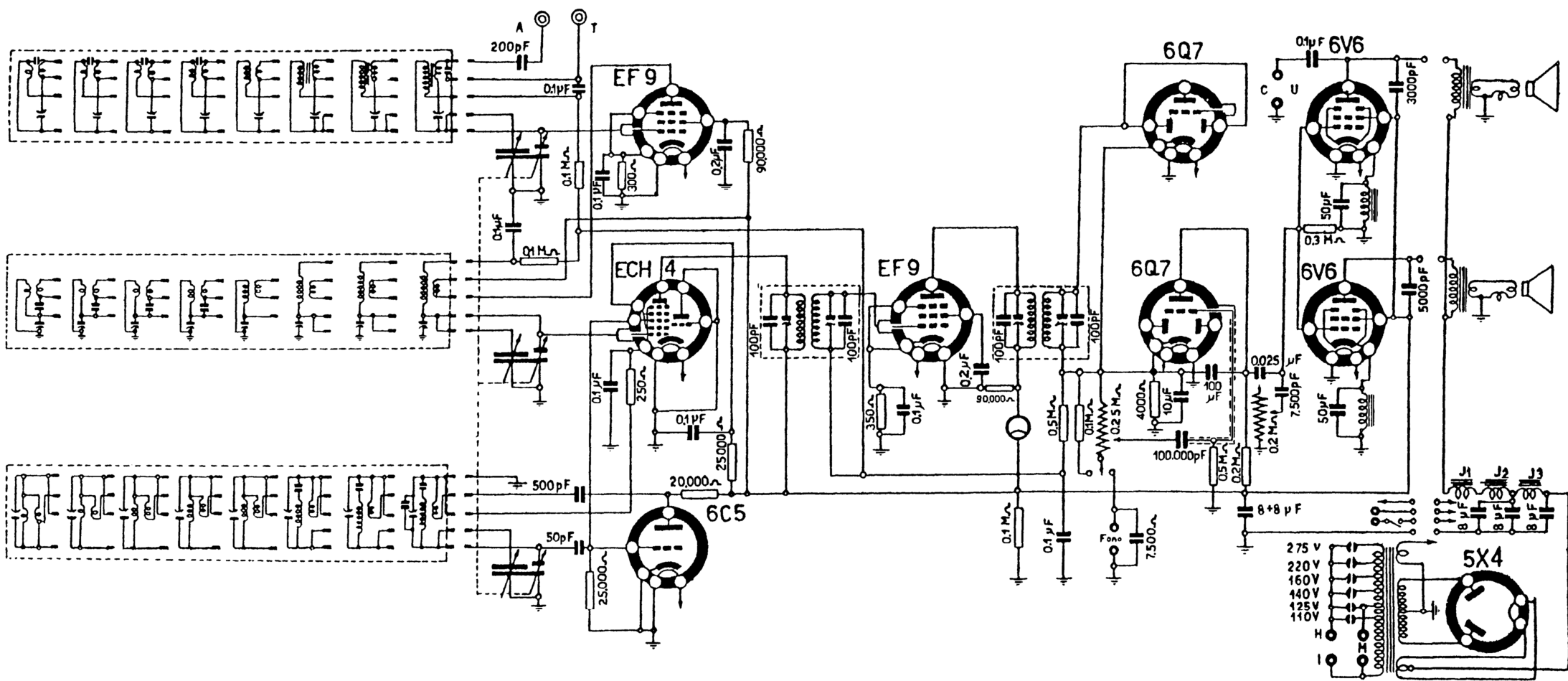
16 - IMCA RADIO - MOD. IF 92S SERIE MULTIGAMMA IV. Una gamma onde lunghe, due gamme onde medie, quattro gamme onde corte. Conversione di frequenza con ECH4 mescolatrice e 6C5 oscillatrice separata. Potenza d'uscita: 12 watt. Media frequenza: 467 kc/s.
